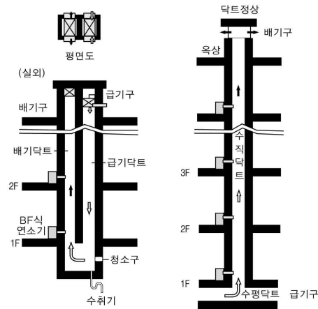
그림 B3.2.3.3.6① SE 및 U덕트의 설치 예시
