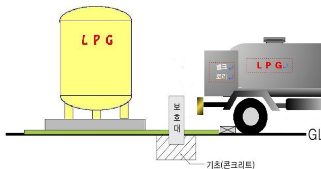
그림 2.3.3.4(5) 보호대 설치방법
