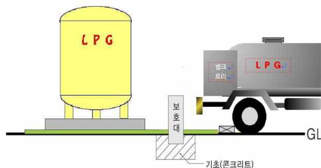
그림 2.3.3.4(5) 보호대 설치방법
