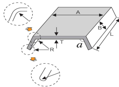
그림 2.5.7.5.3 보호판의 치수
