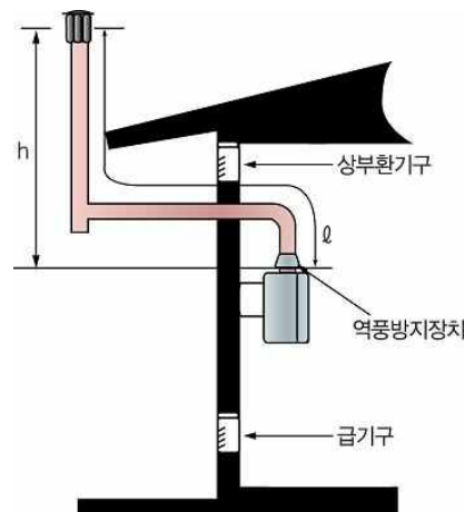
그림 2.7.1.3.1(1) 배기통의 높이
