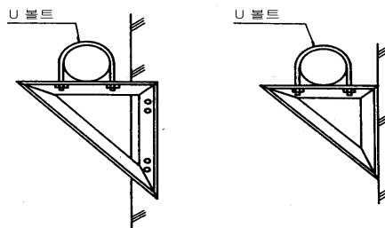
(a) 브라켓지지
