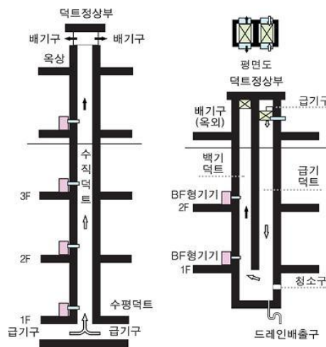
그림 2.7.1.4.2(3) SE 및 U 덕트 설치 예시
