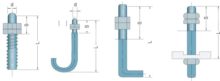
그림 2.2.3.3 앵커보울트의 치수표시
