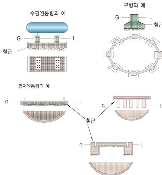
그림 2.2.2.3 저장탱크의 수평기초면
