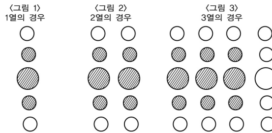
그림 2.9.9.1.4 온도상승방지설비 능력산정기준
