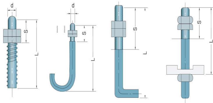
그림 2.2.3.3 앵커보울트의 치수표시
