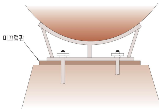
그림 2.2.3.5 미끄럼판의 설치방법
