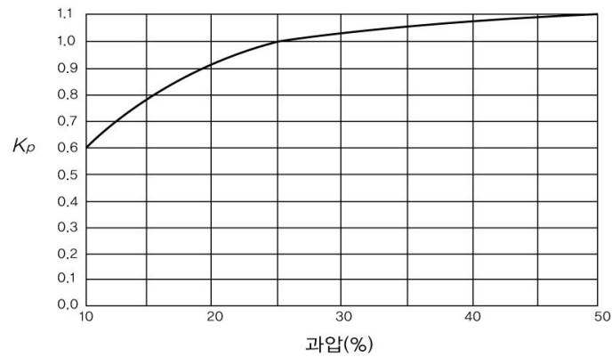
그림 2.7.1.4(2)⑧ 과압보정계수
