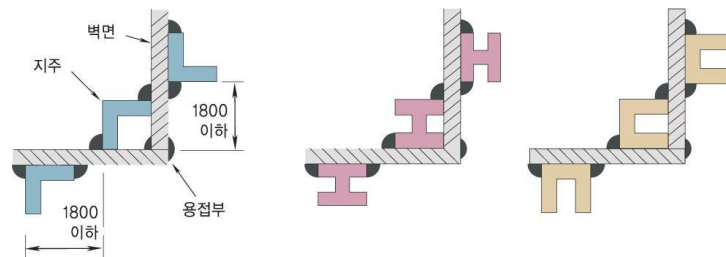
그림 2.8.2.3.4 지주의 설치방법
