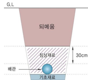
그림 2.5.8.2.5 되메움 구조
