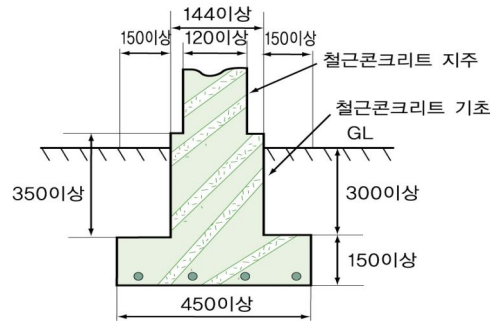
그림 2.8.2.1 철근콘크리트 방호벽의 설치 예
