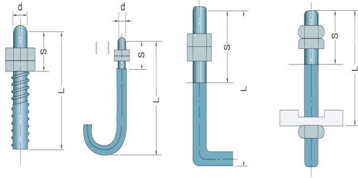
그림 2.2.3.3 앵커보울트의 치수표시
