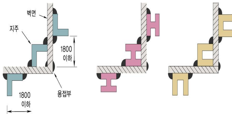
그림 2.8.2.3.4 지주의 설치방법
