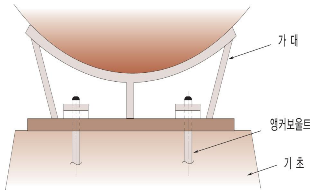
그림 2.2.3.4 앵커보울트의 고정방법
