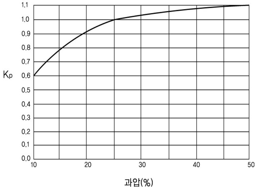
그림 2.7.1.4.2③ 과압보정계수
