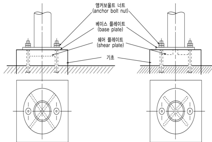
그림 2.2.3.6 구형저장탱크 지주와 기초에 앵커볼트 체결방법
