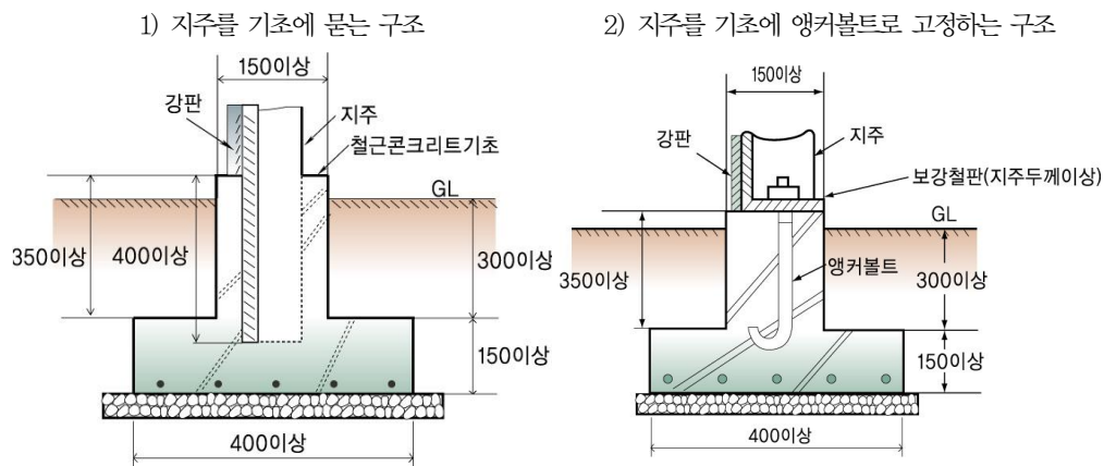
그림 2.8.2.3.6 강판제 방호벽의 고정방법 예
