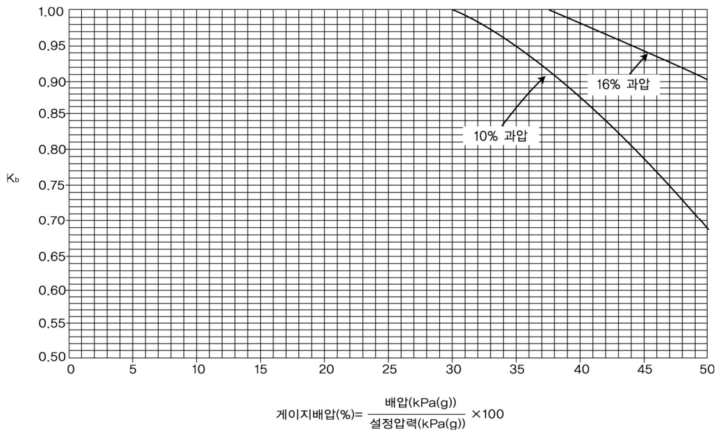
그림 2.6.1.4② 밸런스 밸로우즈형 안전밸브 배압보정계수
