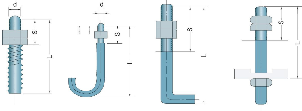
그림 2.2.3.3 앵커보울트의 치수표시
