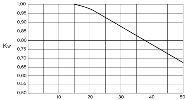
그림 2.6.1.4⑤ 아음속계수
