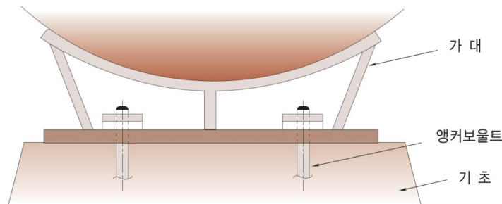
그림 2.2.3.4 앵커보울트의 고정방법
