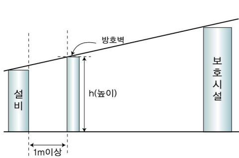
그림 2.7.2.1.2① 방호벽 설치예(측면도)
