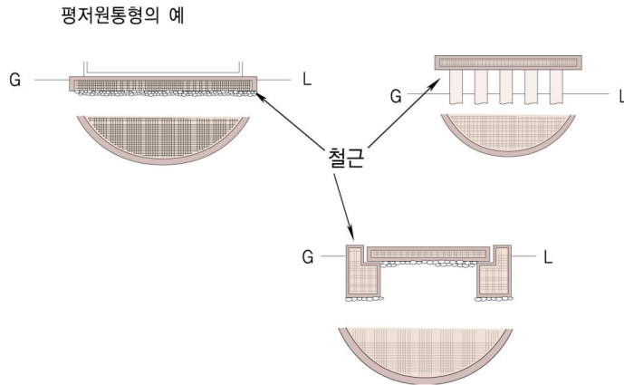
그림 2.2.2.6 저장탱크의 수평기초면
