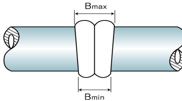
그림 2.5.4.1.4② 비드폭의 최소 및 최대치 표 2.5.4.1.4 호칭지름에 따른 비드폭
