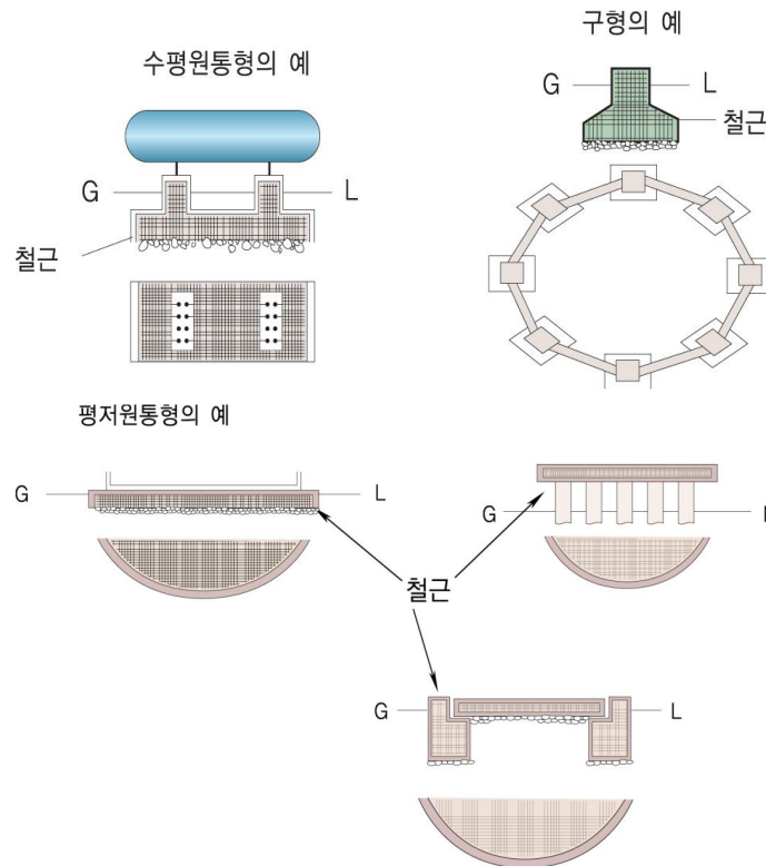
그림 2.2.2.6 저장탱크의 수평기초면
