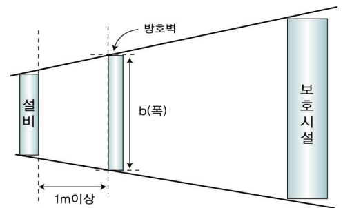
그림 2.7.2.1.2② 방호벽 설치예(평면도)
