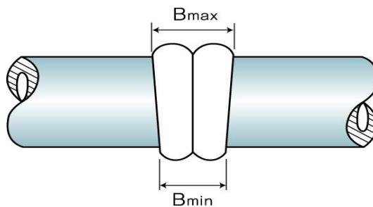
그림 2.5.4.1.4② 비드폭의 최소 및 최대치
