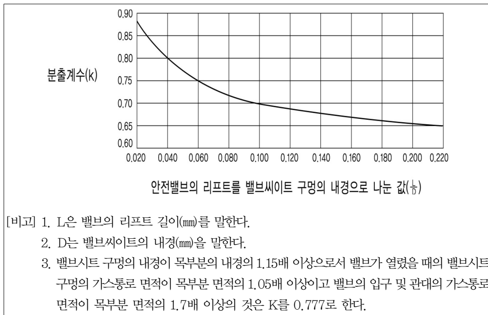
그림 2.6.1.1.4 분출계수
