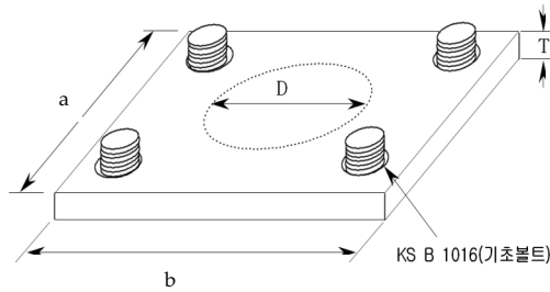
그림 2.3.3.2.35-3-2 강판제 보호대의 방화대 설치 방법
