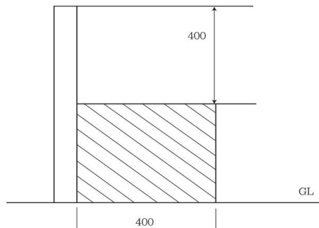
그림 2.7.2.2.4 보조벽의 높이
