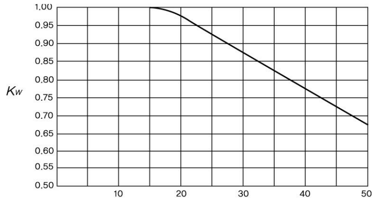
그림 2.6.1.4(2)⑤ 아음속계수
