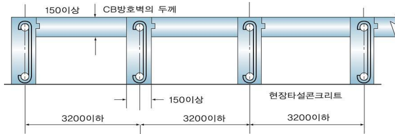
그림 2.7.2.2.3 보조벽의 배치
