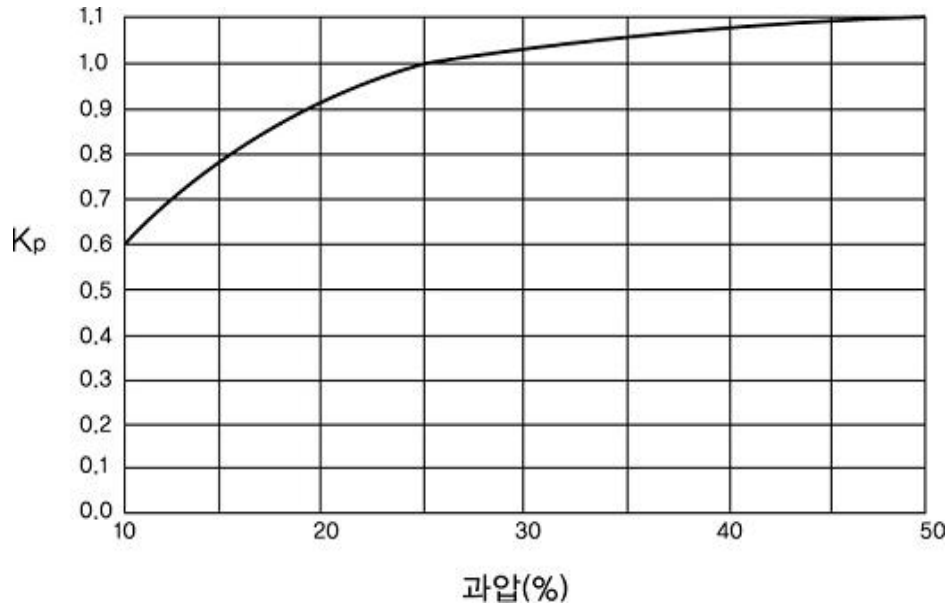
그림 2.6.1.4⑧ 과압보정계수
