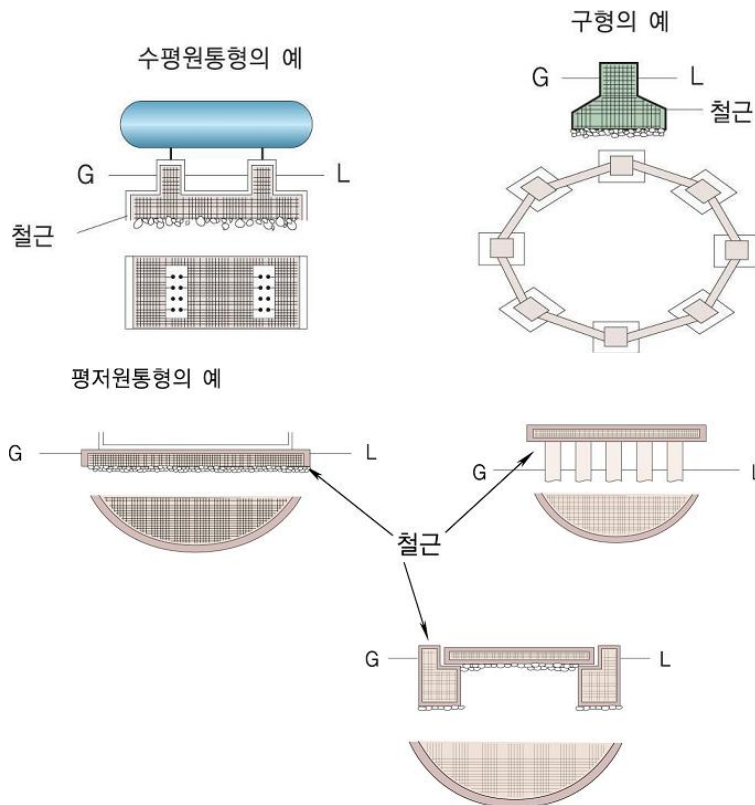
그림 2.2.2.3 저장탱크의 수평기초면
