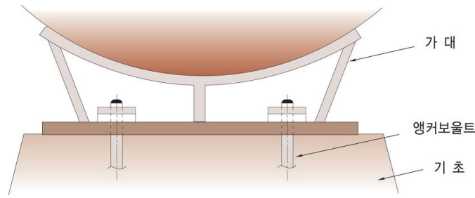
그림 2.2.3.4 앵커보울트의 고정방법
