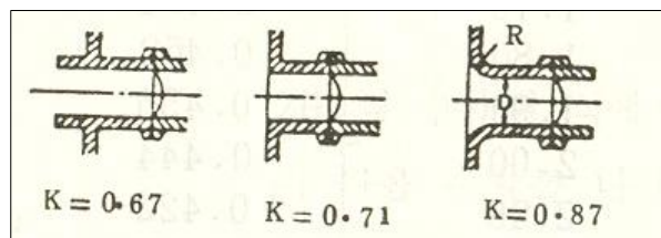
그림 A3.2(1)② 파열판의 분출계수
