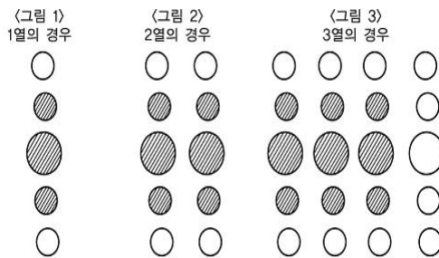
주) 사선 친 부분의 저장탱크가 대대표면적이 됨. 그림 2.7.9.1.4 온도상승방지설비 능력 산정 기준
