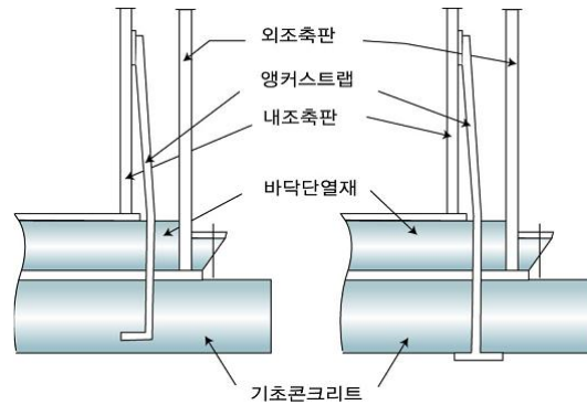
그림 2.2.3.7 평저형 저장탱크의 앵커스트립 설치방법
