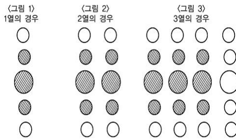
주) 사선 친 부분의 저장탱크가 대대표면적이 됨. 그림 2.7.9.1.4 온도상승방지설비 능력 산정 기준
