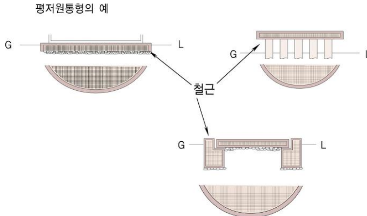
그림 2.2.2.3 저장탱크의 수평기초면
