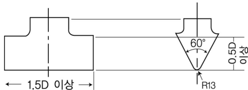
(단위 mm) 그림 4.4.2.2.1(2)③ 압괴시험용 강제썩기
