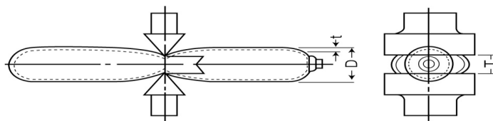
(단위 mm) 그림 4.4.2.2.1(2)③ 압괴시험용 강제썩기
