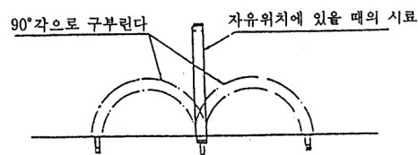
그림 3.8.1.3 호스의 내한성능시험시 급힘방법
