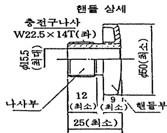
그림 3.4.5 조정기에 연결하는 이음쇠의 치수
