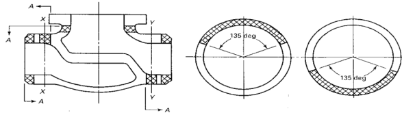
< 볼트체결식 덮개형 글로브밸브 몸통 >
