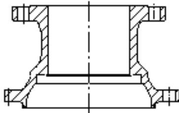
그림 3.8.2.2.1① 볼밸브 방사선투과시험 부위(예시) (개정 12.12.28)
