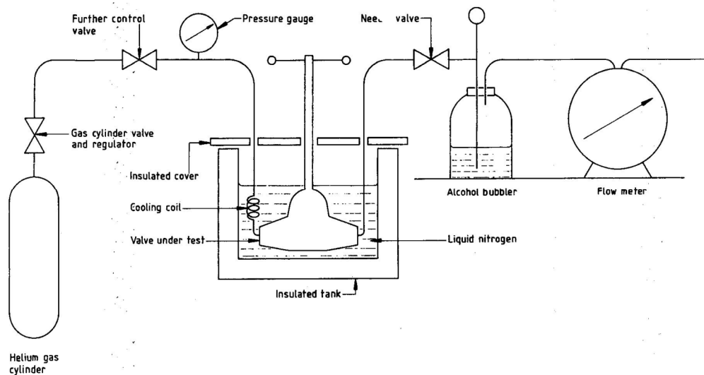
그림 3.8.1.2.4 초저온밸브 기밀시험(예시)
