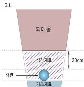
그림 2.5.7.5.5 배관의 매설방법
