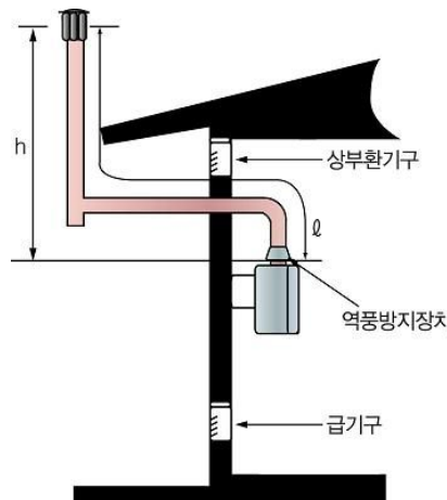
그림 2.7.1.3.1(1) 배기통의 높이
