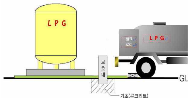
그림 2.3.3.4(5) 보호대 설치방법
