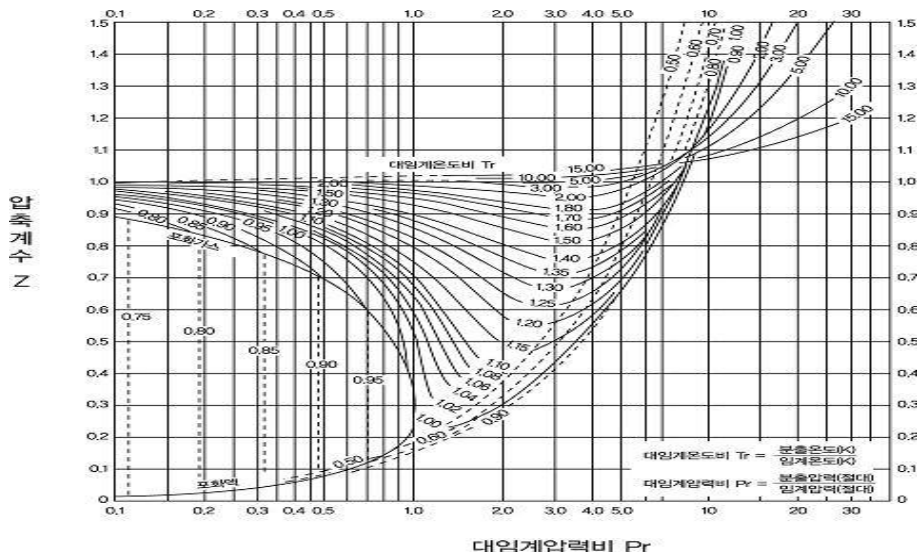
그림 2.8.1.4.1(2)④ 압축계수
