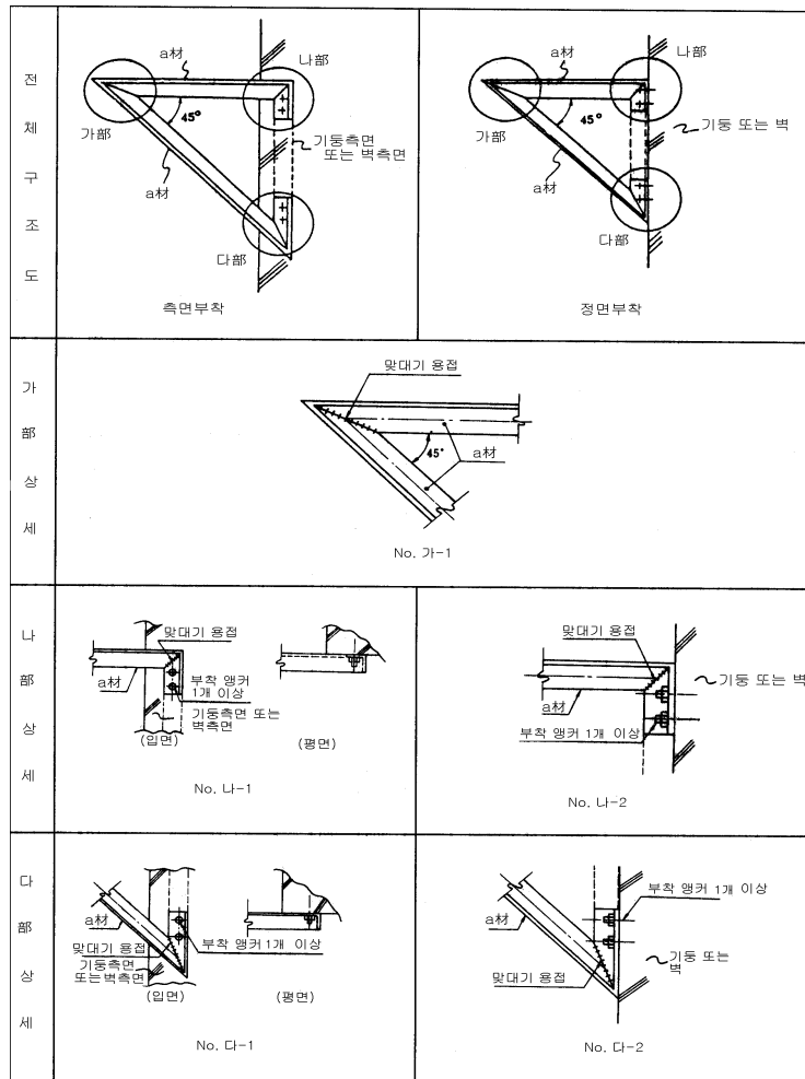
그림 F9.4 횡자관 내진지지구 상세도 및 조립요령
