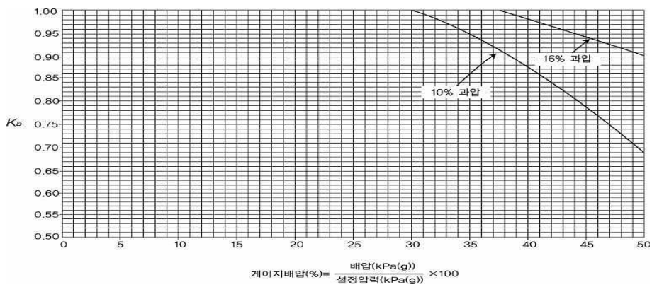
그림 2.8.1.4.1(2)② 밸런스 벨로우즈형 안전밸브 배압보정계수
