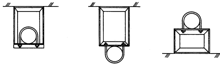
(b) 라멘구조지지
