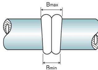
그림 2.5.4.2.2(1)② 용착이음부의 비드폭
