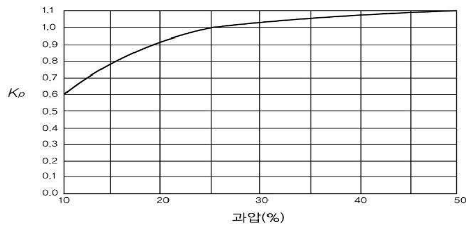
그림 2.8.1.4.1(2)⑧ 과압보정계수
