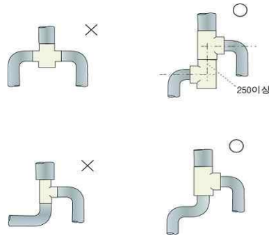
그림 2.7.1.3.1(3) 복합배기통 설치 예
