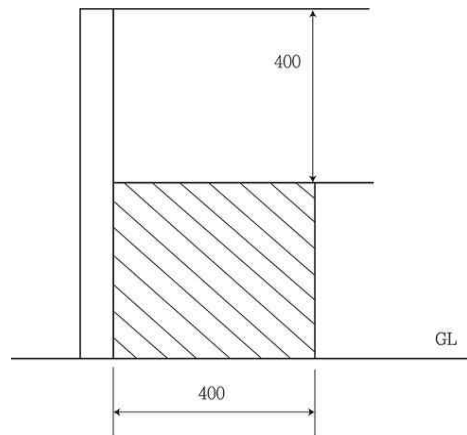
그림 2.9.2.2.3 보조벽의 높이
