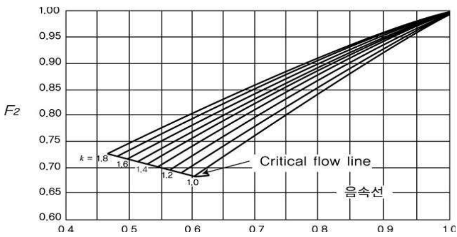
그림 2.8.1.4.1(2)⑤ 아음속계수
