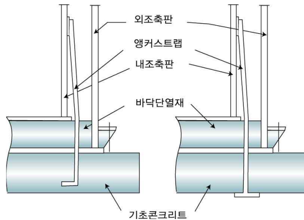
그림 2.2.3.7 평저형 저장탱크의 앵커스트립 설치방법
