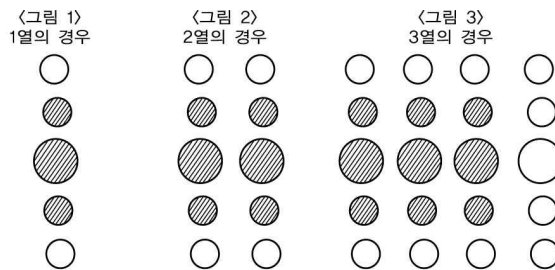
주) 사선 친 부분의 저장탱크가 대서표면적이 됨.
