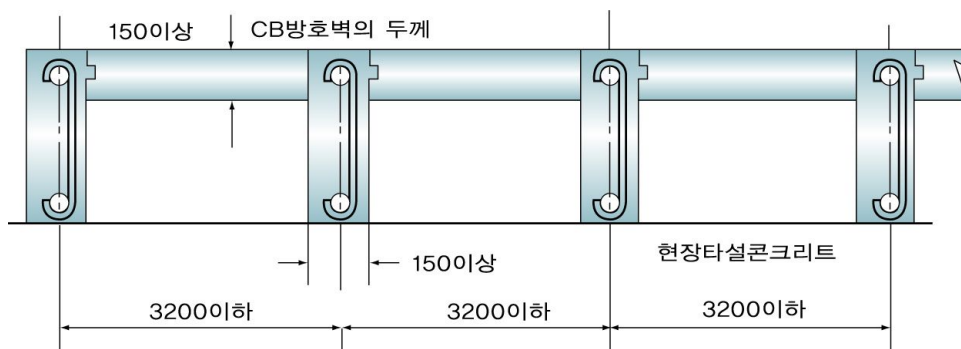
그림 2.8.2.2.2 보조벽의 배치
