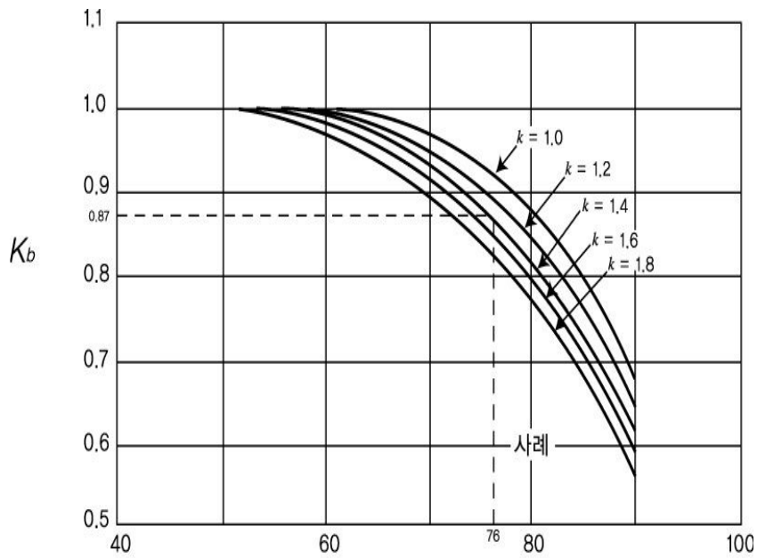
그림 2.7.1.2② 평형밸로우즈형 과압안전장치 배압보정계수
