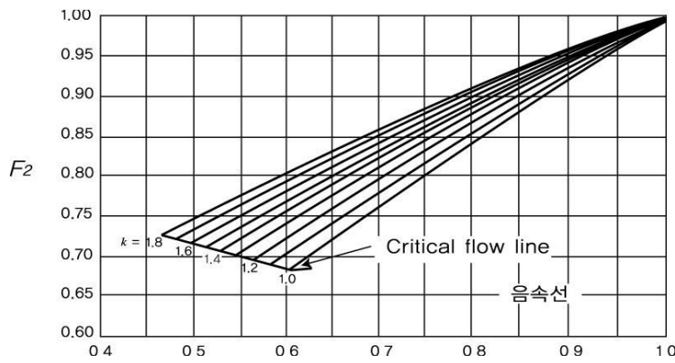
그림 2.7.1.4(2)⑤ 아음속계수
