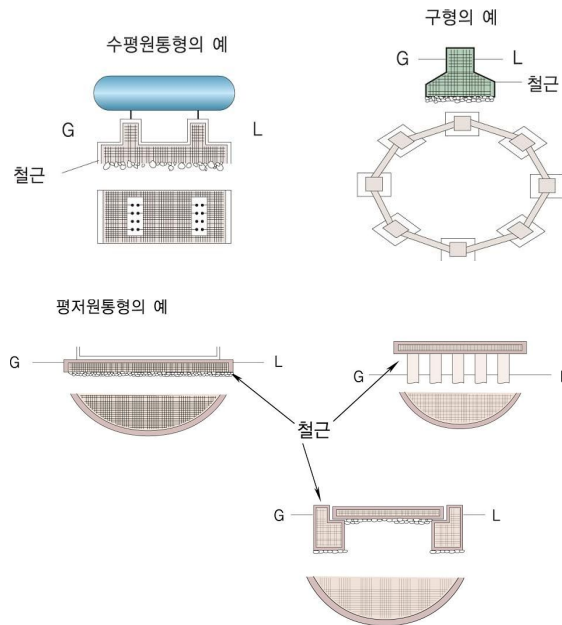
그림 2.2.2.4 저장탱크의 수평기초면
