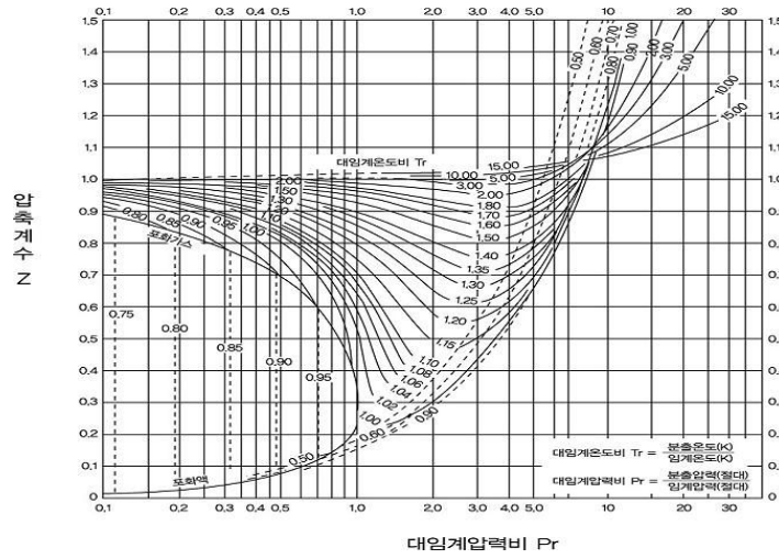
그림 2.7.1.4(2)④ 압축계수
