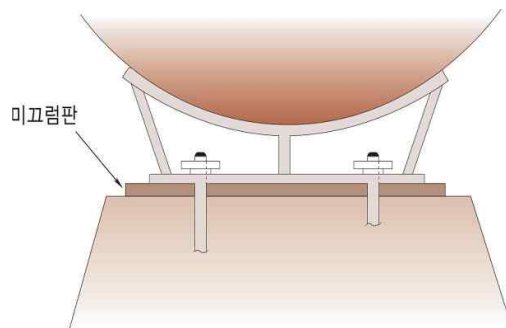
그림 2.2.3.5 미끄럼판의 설치방법
