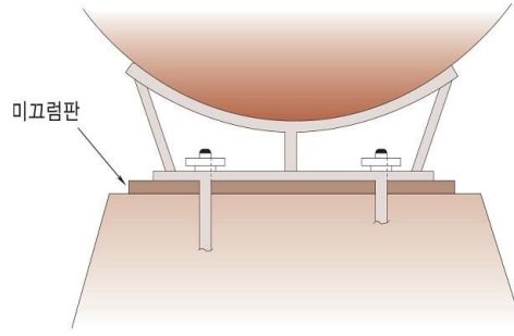
그림 2.2.3.5 미끄럼판의 설치방법
