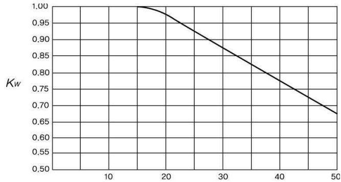
그림 2.6.1.4(2)⑤ 아음속계수
