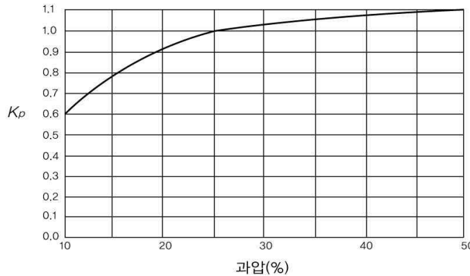
그림 2.6.1.4(2)⑧ 과압보정계수
