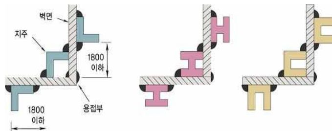
그림 2.7.2.3.4 지주의 설치방법
