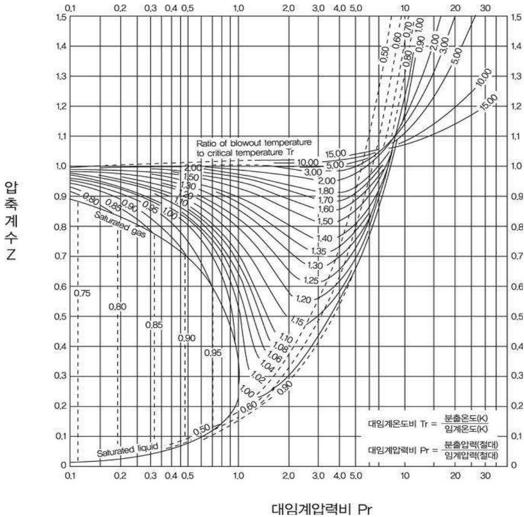
그림 2.6.1.4④ 압축계수
