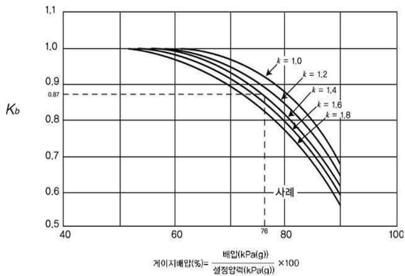
그림 2.6.1.4③ Conventional 안전밸브 배압조정계수
