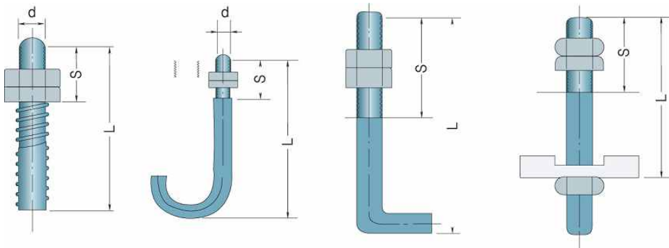
그림 2.2.3.3 앵커보울트의 치수표시
