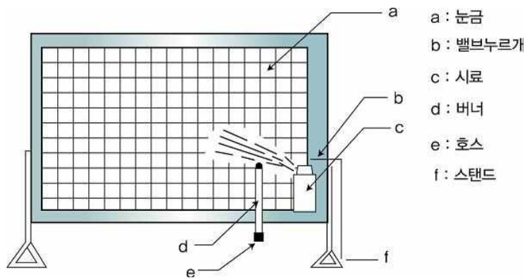
그림 3.2.2.1.2(2) 불꽃 길이 시험장치
