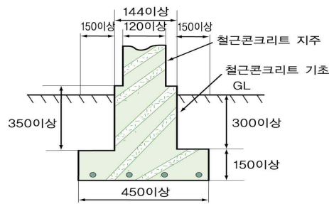
그림 2.7.2.1.2 철근콘크리트제 방호벽 설치예
