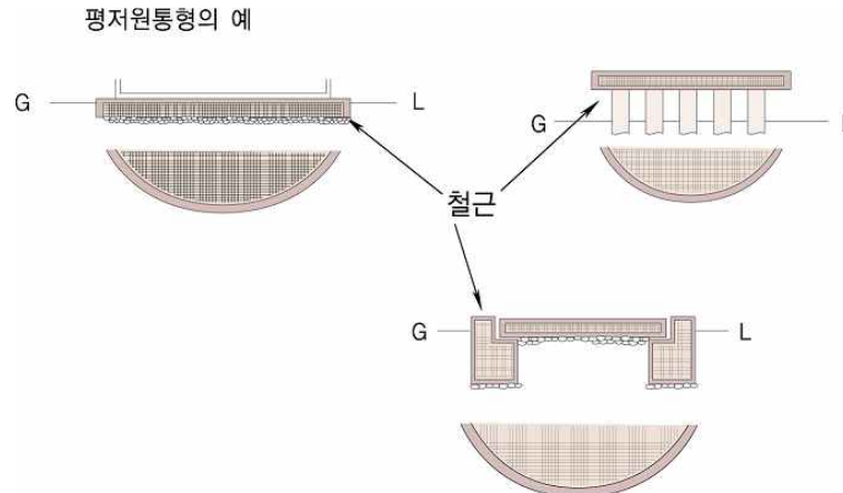
그림 2.2.2.3 저장탱크의 수평기초면
