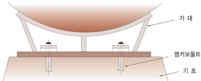
그림 2.2.3.4 앵커보울트의 고정방법
