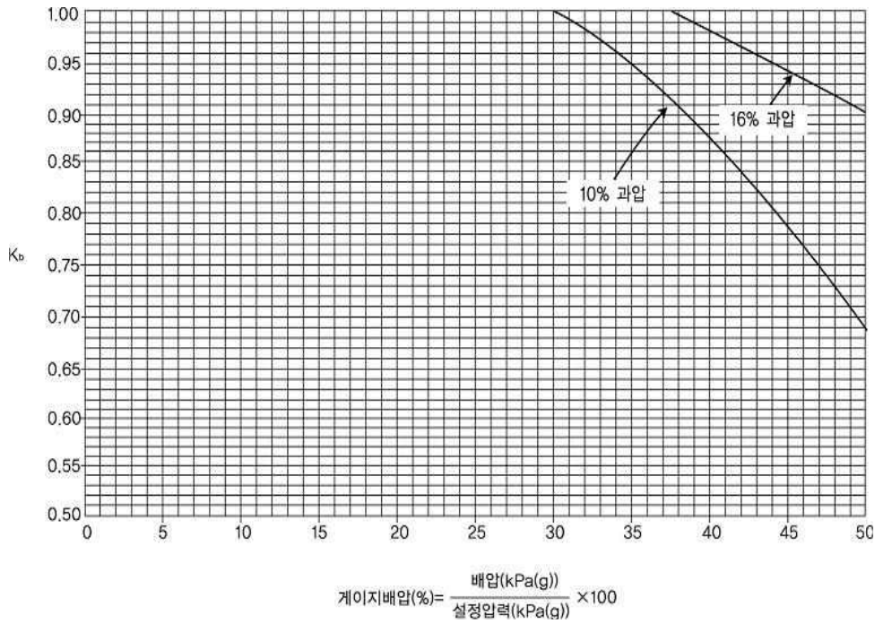
그림 2.6.1.4② 밸런스 벨로우즈형 안전밸브 배압보정계수
