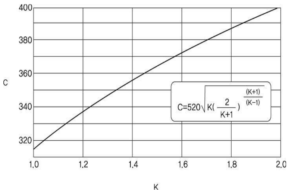
그림 2.6.1.4① 열용량비 k=C_p/C_v
