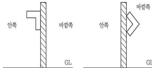
그림 2.7.2.3.2 강판제방호벽의 앵글강 보강
