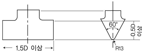
그림 4.4.2.2.1(2)③ 압괴시험용 강제썩기
