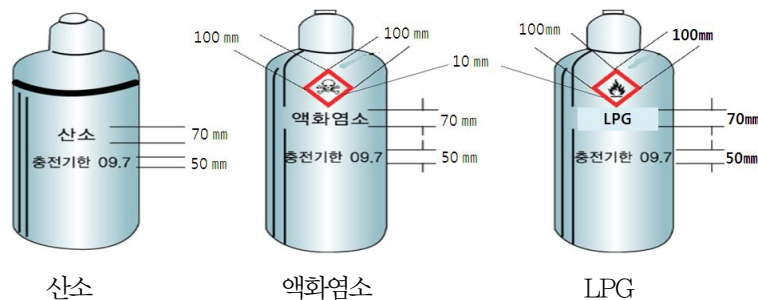
그림 3.12.2.2.2① 일반·공업용 가스용기 문자 크기
