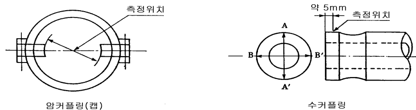
그림 4-1 커플링
