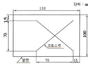
그림 3. 도막의 염수 분무 시험용 시편
