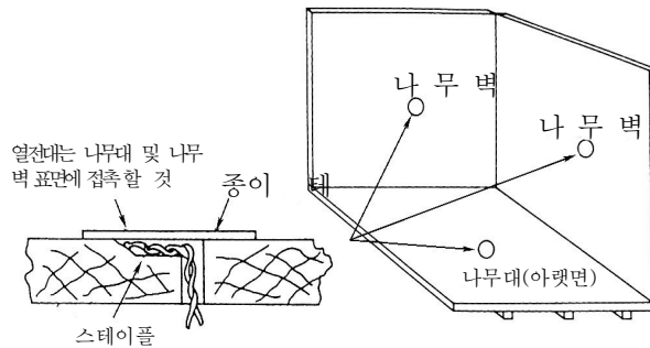
그림 나무대 및 나무벽 표면 온도 측정 장치
