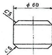
그림 3.4.2.6.1 낙하체의 형상
