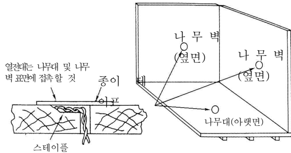
그림 나무대 및 나무벽 표면 온도 측정 장치
