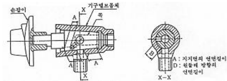
그림 3.2.24.3 콕 구조의 기구 밸브
