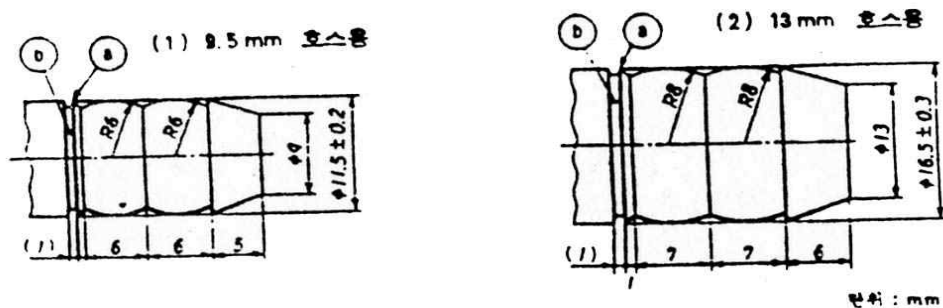
그림 3.2.23.3 호스 접속구의 모양 및 치수
