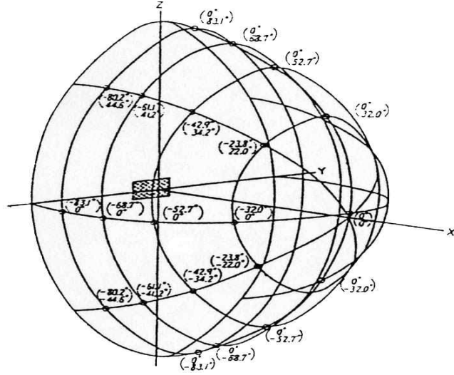
그림 C6 . 방사각도의 측정
