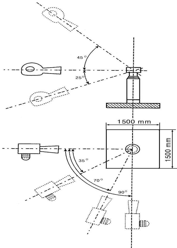
그림 G2. 지붕에 설치될 다기능 보일러 유풀시험장비
