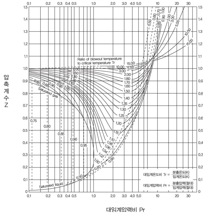
그림 2.6.1.4④ 압축계수
