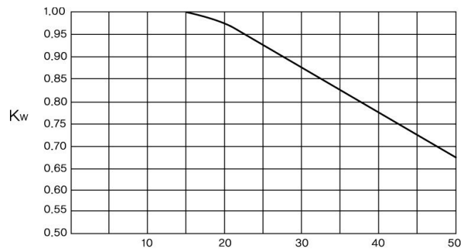
그림 2.6.1.4⑤ 아음속계수
