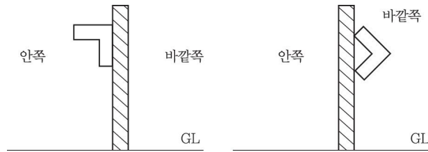
그림 2.7.2.3.2 강관제방호벽의 앵글강 보강
