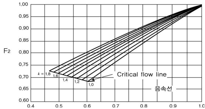
그림 2.6.1.4⑤ 아음속계수
