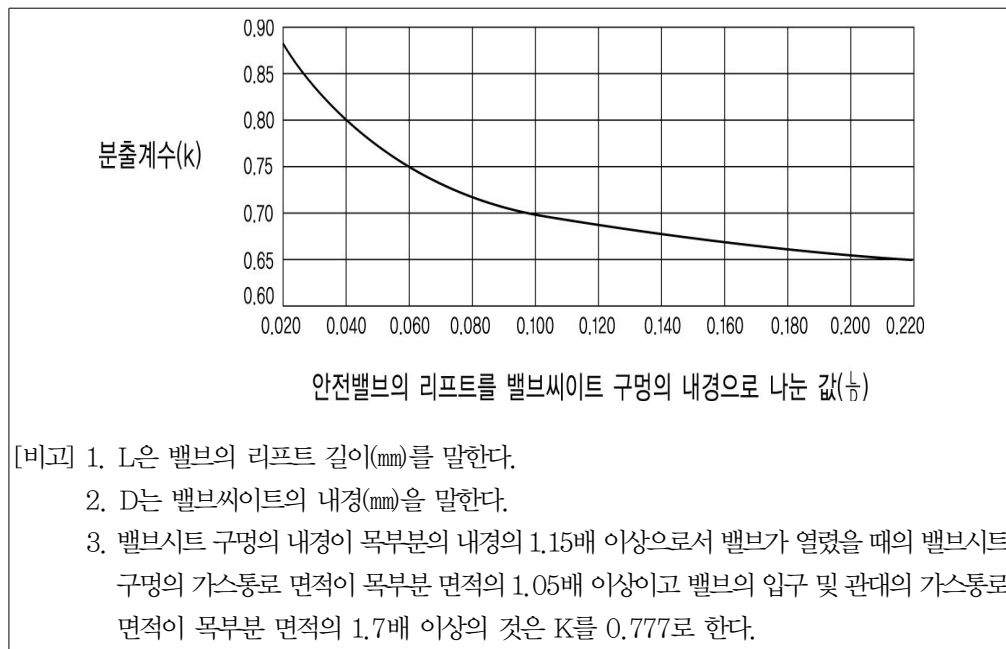
그림 2.6.1.1.4 분출계수
