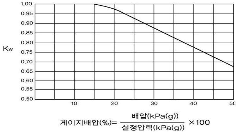
그림 2.6.1.4⑥ 밸런스 벨로우즈형 안전밸브 배압보정계수
