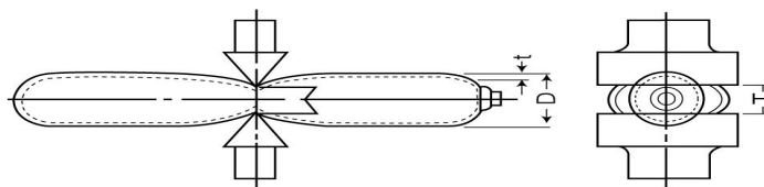
그림 4.4.2.2.1(2)③ 압괴시험용 강제썩기
