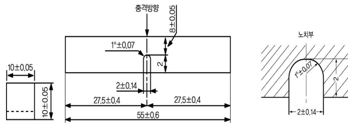
3호시험편 (KS B 0809) (단위 mm) 그림 4.4.2.2.1(2)② 제3호 시험편(KS B 0809)
