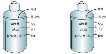
그림 3.12.2.2.2② 의료용 가스 용기 문자 크기
