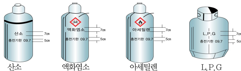
그림 3.12.2.2.2① 일반·공업용 가스용기 문자 크기
