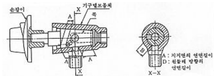
그림 3.2.20.3 록 구조의 기구 밸브
