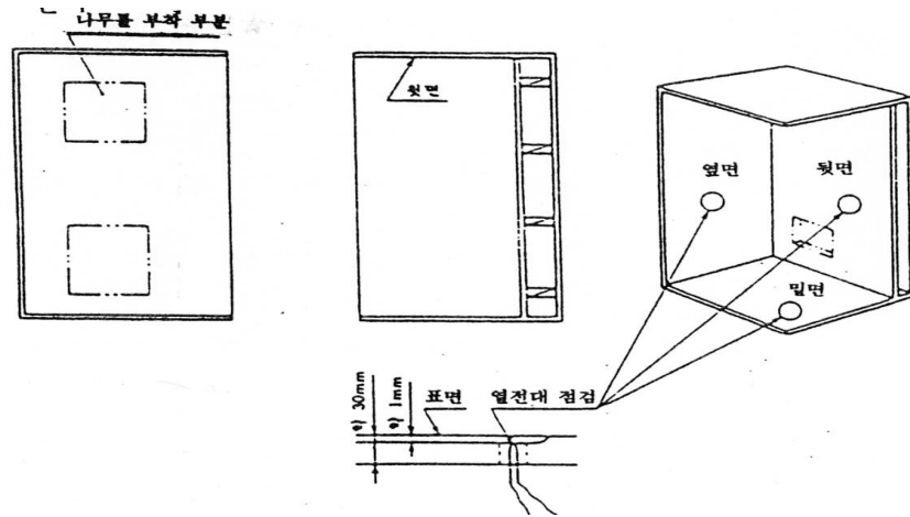
그림 6. 나무대 및 나무벽 표면온도 측정장치
