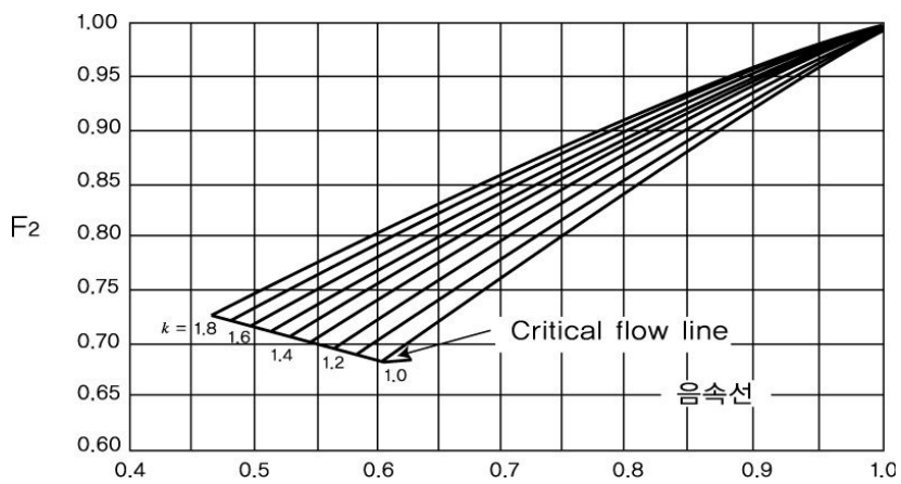
그림 3.4.6.3.1⑤ 아음속계수
