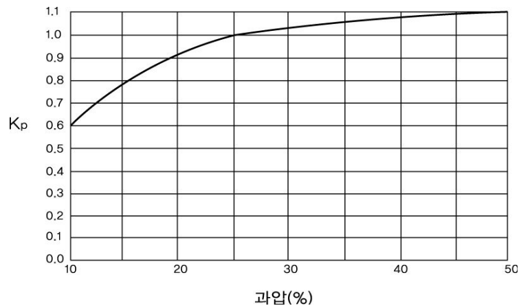
그림 3.4.6.3.1⑧ 과압보정계수
