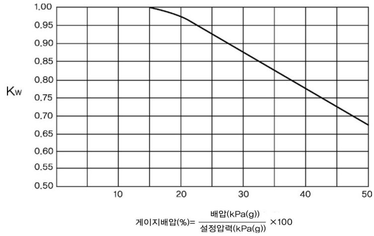
그림 3.4.6.3.1⑥ 밸런스 벨로우즈형 안전밸브 배압보정계수
