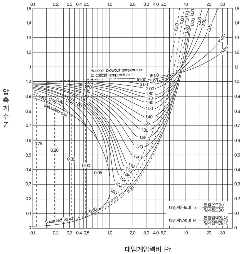
그림 3.4.6.3.1④ 압축계수
