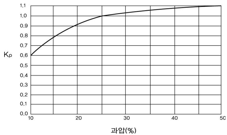
그림 3.4.6.3.1⑧ 과압보정계수
